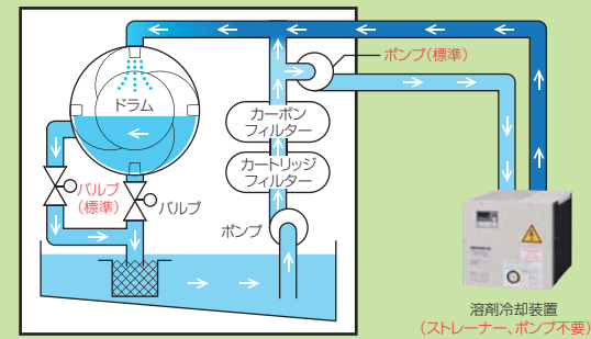
DMIシリーズ配管系統図
