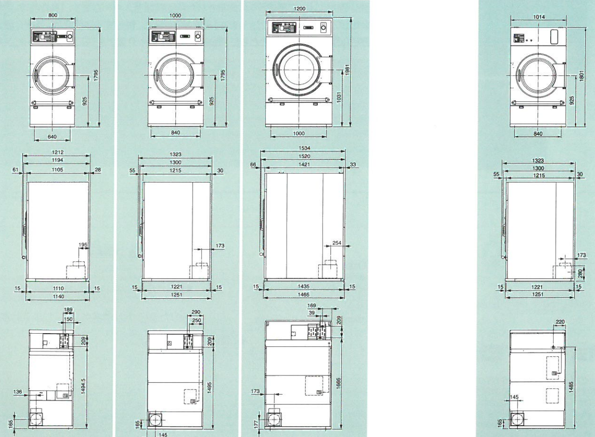
外形寸法図
